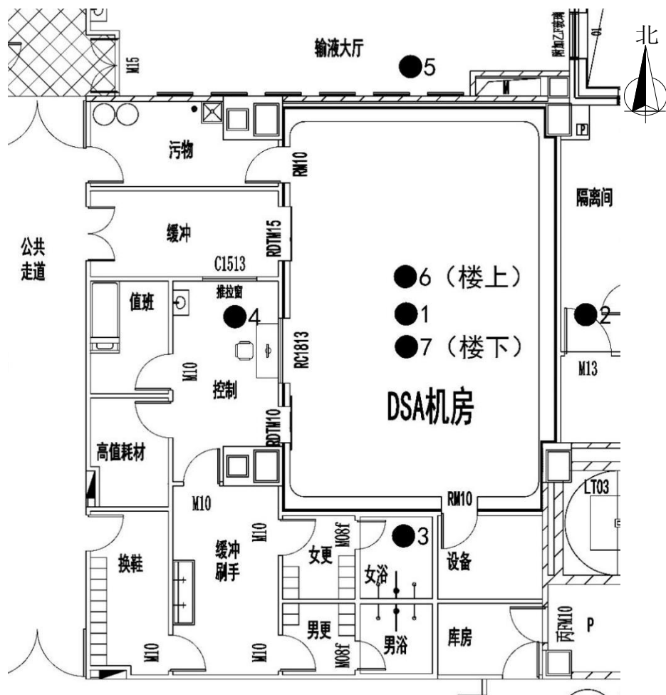
图 8-1 介入 DSA 室周围检测点位图
