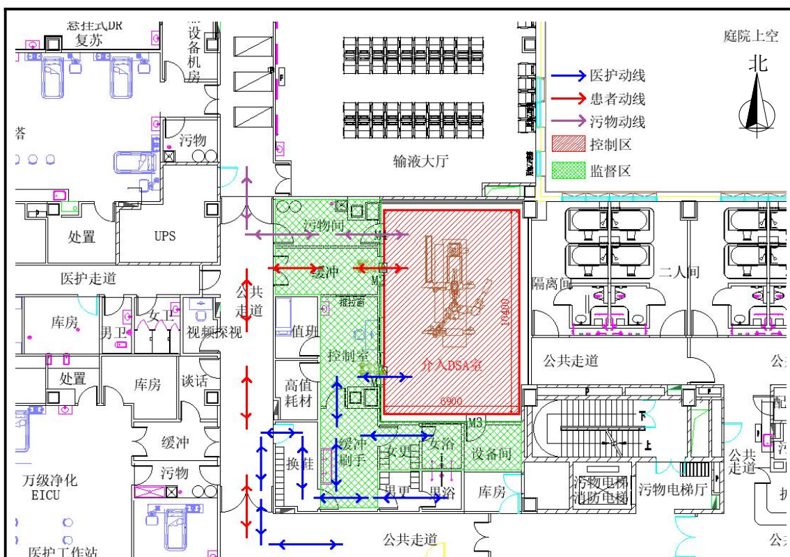
图 11-1 医院介入 DSA 室分区和路由平面布局图
