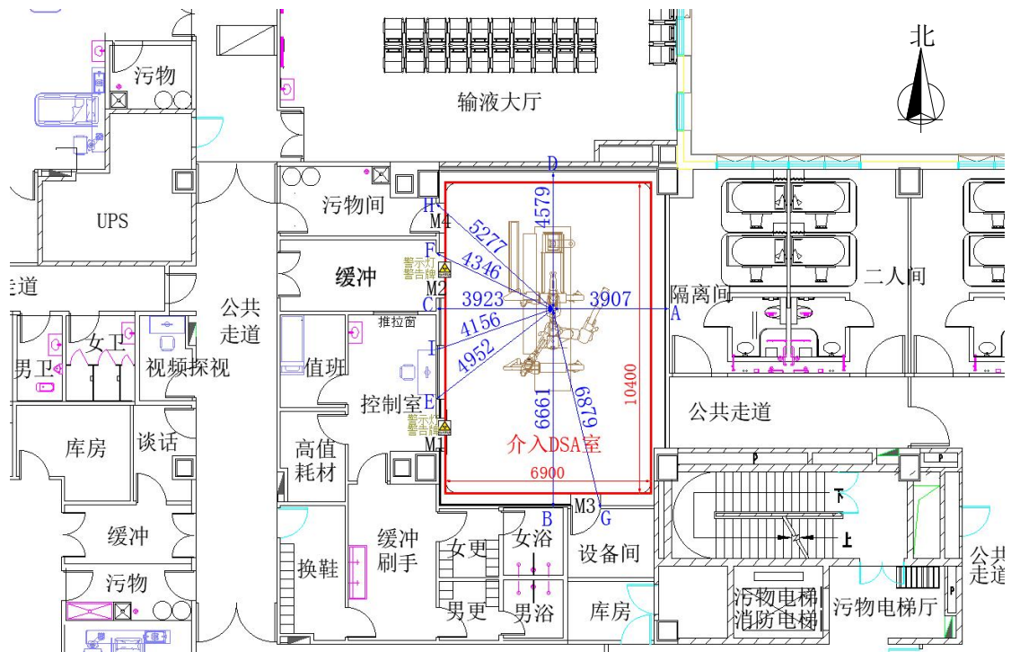
图 11-2 介入 DSA 室估算点位示意图
