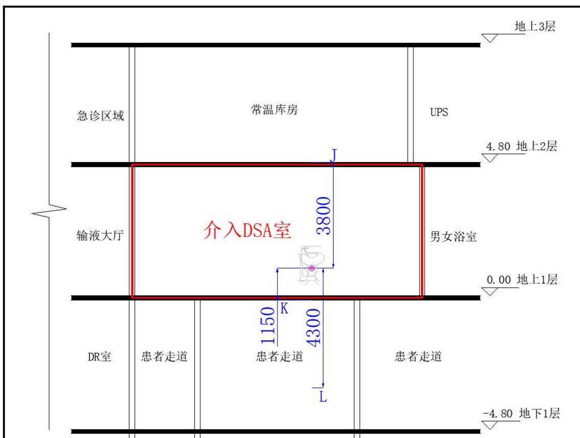
图 11-3 介入 DSA 室楼上、楼下南北向剖面图
