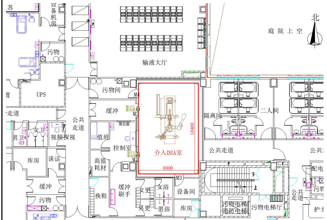
图 7-2 介入 DSA 室四周毗邻关系图
