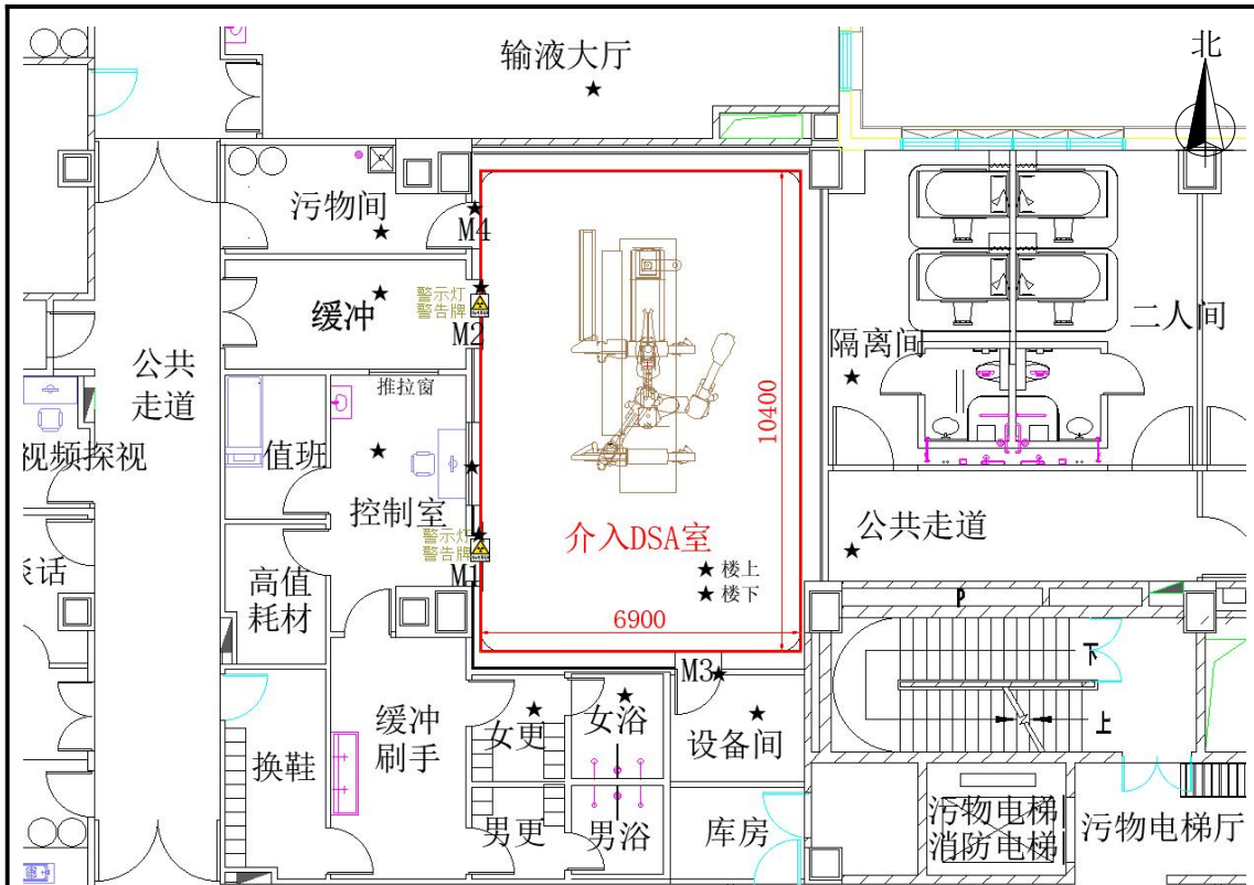
图 12-1 介入 DSA 室周围自行检测点位图（标注★为检测位置）
